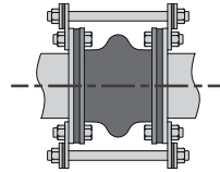
شكل 6.4 - مثال على وصلة مطاطية مع شدادات تحديد
