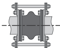
6.4 pav. – Guminės jungties su ribojančiais jungiamaisiais strypais pavyzdys
