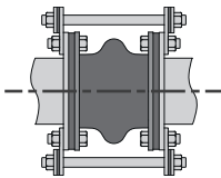
Kuva 6.4 - Esimerkki kumiiliitoksesta, jossa on rajoittavat tasaustangot
