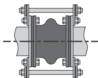
Fig. 6.4 - Esempio di giunto in gomma con tiranti di limitazione
