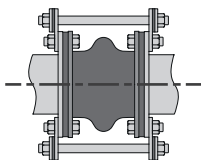
Fig. 6.4 - Exemplu de cuplaj din cauciuc cu tiranți de limitare
