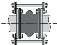
Afb. 6.4 - Voorbeeld van rubberen koppeling met begrenzende trekstangen
