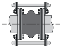
6.4. attēls – Gumijas savienojuma piemērs ar ierobežojošiem savienotājstieniem.
