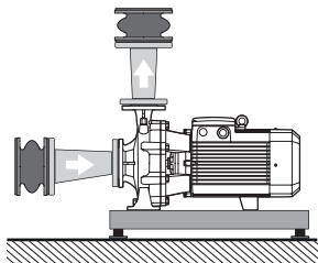
Abb. 6.3 – Beispiel für Installation zur Reduzierung von Vibrationen und Geräuschen
