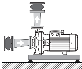
Fig. 6.3 - Eksempel på installation til at reducere vibrationer og støj
