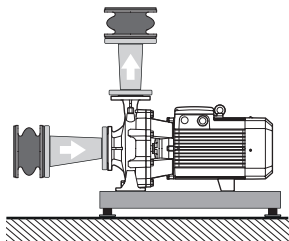
Afb. 6.3 - Installatievoorbeeld om trillingen en lawaai te verminderen
