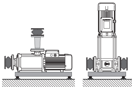
Sl. 6.5 – Primer ugradnje za smanjenje vibracija i buke
