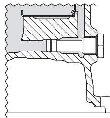
Obr. 7.3 – Vypúšťacia zátka D
