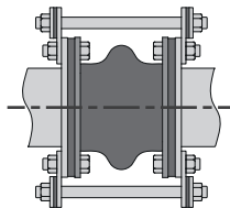
Joonis 6.6 - Näide piiravate tõmmitsatega kummist liigendist
