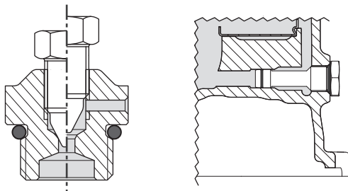
Joonis 7.2. ventilatsioonikork V Joonis 7.3. tühjendustoru kork D
