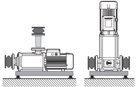
شكل 6.5 – مثال على التركيب لتقليل الاهتزازات والضوضاء
