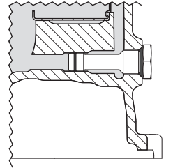
شكل 7.2 - سدادة التنفيس V
