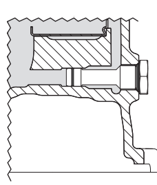
Fig. 7.3 – Avtappningsplugg D
