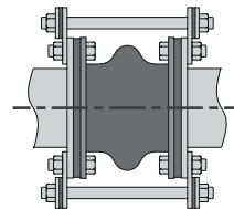
Εικ. 6.6 – Παράδειγμα συνδέσμου από καουτσούκ με ράβδους περιορισμού
