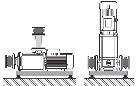
Fig. 6.5 – Exemple d'installation visant à réduire les vibrations et le bruit
