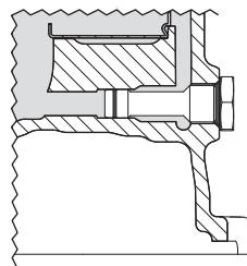
Fig. 7.3 – Tapón de vaciado D
