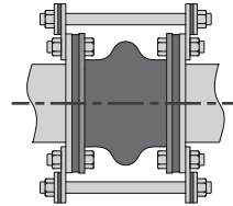
Fig. 6.6 – Ejemplo de junta de caucho con tirantes de limitación
