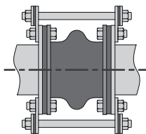
Fig. 6.6 – Eksempel på gummifuge med fastholdelsesstænger
