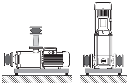
Fig. 6.5 – Exemplu de instalare pentru reducerea vibrațiilor și a zgomotului
