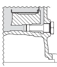
Sl. 7.3 – Čep za ispuštanje D
