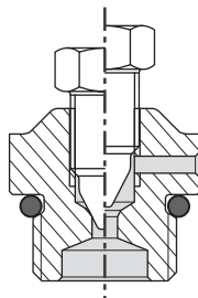
Sl. 7.2 – Odzračevalni vijak
