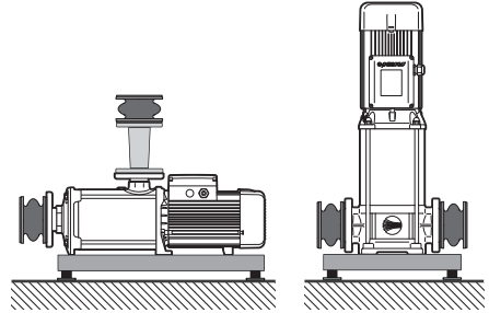
6.5. ábra – Beépítési példa a rezgések és a zaj csökkentésére
