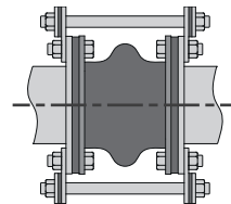
Abb. 6.6 – Beispiel für Gummikompensator mit Zugstangen
