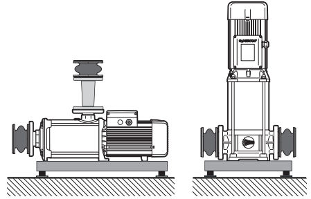
Fig. 6.5 – Ejemplo de instalación para reducir las vibraciones y el ruido
