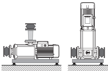
Rys. 6.5 – Przykład instalacji w celu zmniejszenia wibracji i hałasu
