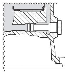
Εικ. 7.3 – Τάπα αποστράγγισης D
