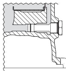
Obr. 7.3 – Vypouštěcí zátku D
