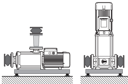
Afb. 6.5 – Installatievoorbeeld om trillingen en lawaai te verminderen
