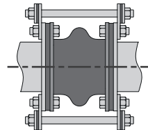
Kuva 6.6 – Esimerkki kumiliitoksesta, jossa on rajoittavat tasaustangot
