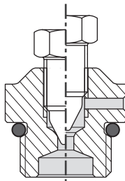
Fig. 7.2 – Bușon de aerisire V
