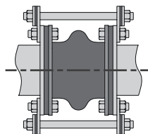
Fig. 6.6 – Exemplo de junta de borracha com tirantes de limitação
