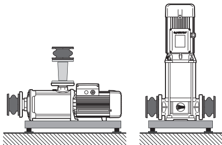
Fig. 6.5 – Esempio di installazione per ridurre vibrazioni e rumore
