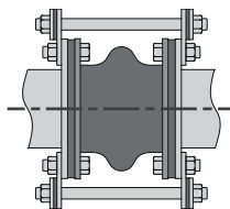
Afb. 6.6 – Voorbeeld van rubberen koppeling begrenzendende trekstangen
