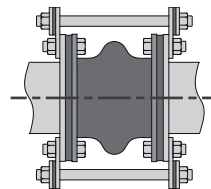
Фиг. 6.6 - Пример за гумено съединение със задържащи пръти
