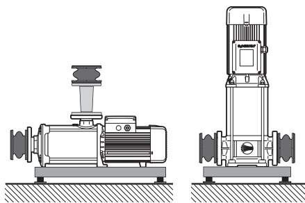
Fig. 6.5 – Eksempel på installation til at reducere vibrationer og støj
