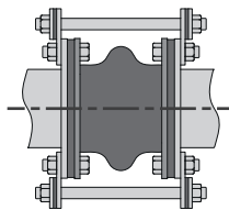
6.6 pav. – Guminės jungties su ribojančiais jungiamaisiais strypais pavyzdys
