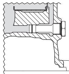
Abb. 7.3 – Ablassstopfen D
