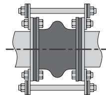
Fig. 6.6 – Exemple de raccord en caoutchouc avec tiges de maintien
