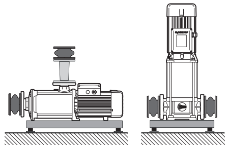
Фиг. 6.5 – Пример за монтаж за намаляване на вибрациите и шума
