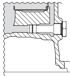
7.3. ábra – D leeresztőcsavar
