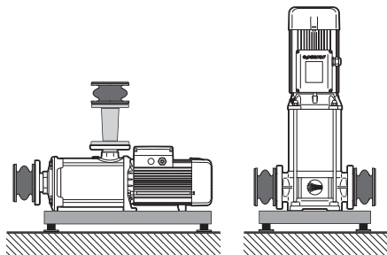
Sl. 6.5 – Primer montaže za zmanjšanje vibracij in hrupa
