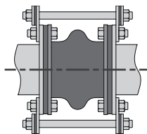
Rys. 6.6 – Przykład złącza elastycznego ze ściągami ograniczającymi
