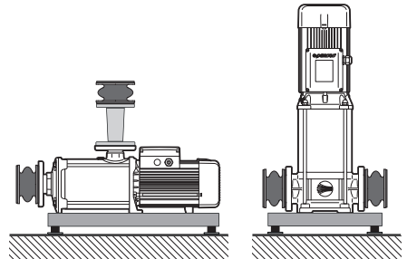
Εικ. 6.5 – Παράδειγμα εγκατάστασης για τη μείωση δονήσεων και θορύβου
