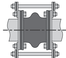
شكل 6.6 – مثال على وصلة مطاطية مع شدادات تحديد
