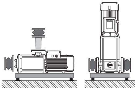
Fig. 6.5 – Exemplo de instalação para reduzir vibrações e ruído
