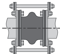
Sl. 6.6 – Primer gumenog spoja sa graničnim vučnim šipkama
