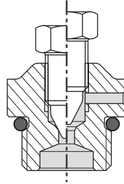
شكل 7.3 - سدادة الصرف D
