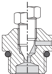
Afb. 7.2 – Ontluchtingsdop
