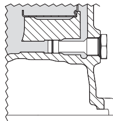
Rys. 7.3 – Korek spustowy D
