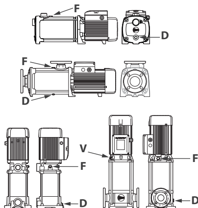
7.1. attēls F = uzpildes vāciņš D = iztukšošanas aizbāznis V = ventilācijas kontaktdakša
