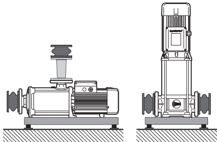
Joonis 6.5. Näide vibratsiooni ja müra vähendava paigalduse kohta
