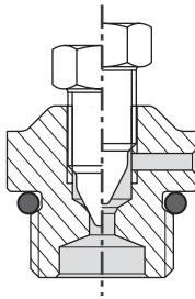
7.2. ábra – V szellőzőcsavar
