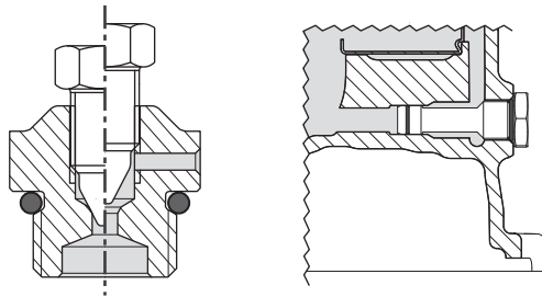
איור 7.2 – פקק אוורור V איור 7.3 – פקק ניקוז D
