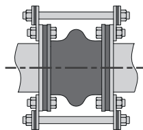
Sl. 6.6 – Primer gumijastega spoja z omejevalnimi vezmi
