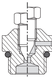
Sl. 7.2 – čep za odzračivanje V
