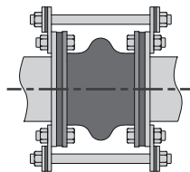
Fig. 6.6 – Esempio di giunto in gomma con tiranti di limitazione
