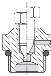
Εικ. 7.2 – Τάπα εξερισμού V
