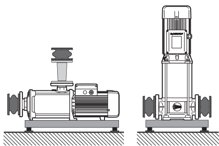
Fig. 6.5 – Exempel på installation för att minska vibrationer och buller
