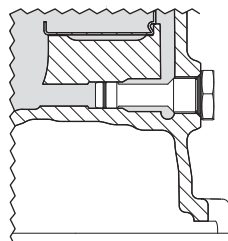
Sl. 7.3 – Vijak za praznjenje D
