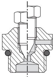
Fig. 7.2 – Udluftningsprop V
