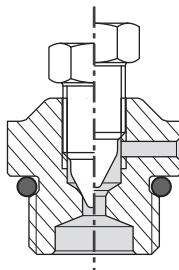
Фиг. 7.2 – Тапа за обезвъздушаване V Фиг. 7.3 – Тапата за източване D
