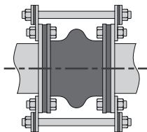
Fig. 6.6 – Exemplu de cuplaj din cauciuc cu tiranți de limitare
