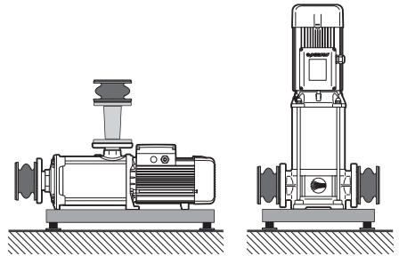
Abb. 6.5 – Beispiel für Installation zur Reduzierung von Vibrationen und Geräuschen
