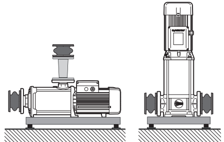
Kuva 6.5 – Asennusesimerkki tärinän ja melun vähentämiseksi
