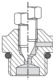
Fig. 7.2 – Tapón de ventilación V
