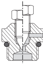
Fig. 7.2 – Tampão de ventilação V
