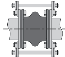
6.6. ábra – Példa gumicsuklóra határoló rúddal
