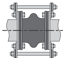
Obr. 6.6 - Příklad gumového kloubu s omezovacími táhly
