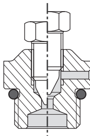
Abb. 7.2 – Entlüftungsstopfen V
