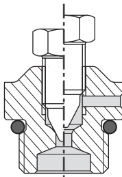
Obr. 7.2 – Odvzdušňovacia zátka V
