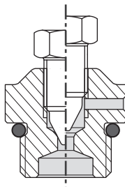
Fig. 7.2 – Bouchon d'évent V
