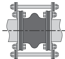
6.6. attēls – Gumijas savienojuma piemērs ar ierobežojošiem savienotājstieniem.
