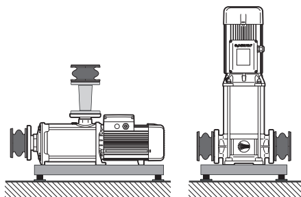
Obr. 6.5 - Příklad instalace pro snížení vibrací a hluku
