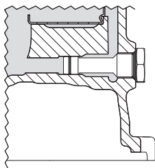
Fig. 7.3 – Afløbsstuds D
