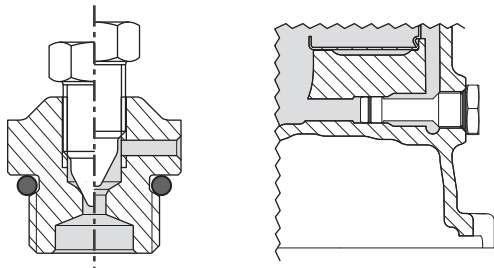
7.2. attēls – Ventilācijas aizbāznis V 7.3. attēls – Iztukšošanas aizbāznis D
