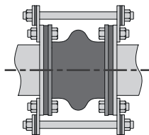
Sl. 6.6 – primjer gumenog spoja s graničnim šipkama
