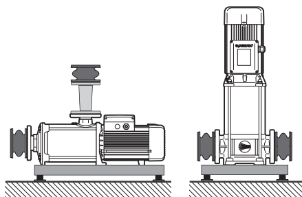
6.5. attēls – Vibrācijas un trokšņa samazināšanas sistēmas piemērs.
