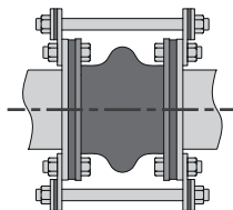
Obr. 6.6 – Příklad gumového spoja s obmedzovacími tiahľami
