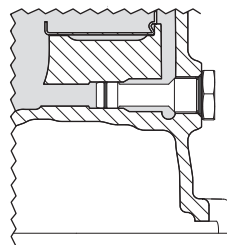
Fig. 7.3 – Tampão de descarga D
