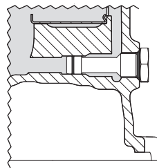
Fig. 7.3 – Bușon de scurgere D
