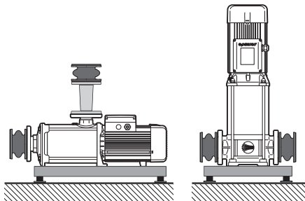
Obr. 6.5 – Příklad inštalácie tlmiacej vibrácie a znižujúcej hluk
