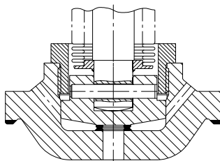
Cône de décharge
