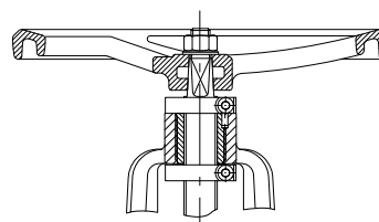
Dispositif de blocage / limiteur de course
