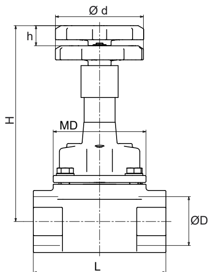
III. 6: Robinet à commande manuelle SISTO-16 à manchons taraudés
