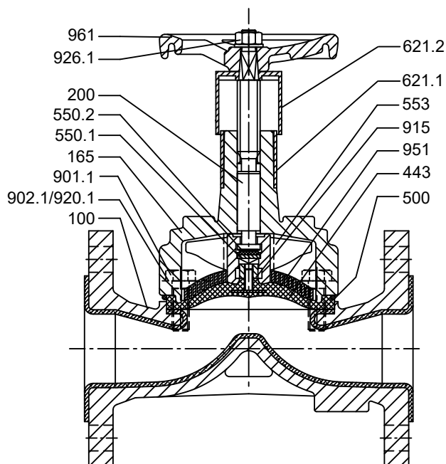
III. 1: Robinet à commande manuelle SISTO-16 avec raccordement à brides
