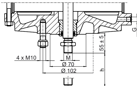
Raccordement à brides F10
