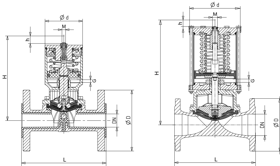
III. 7: Robinets à membrane avec actionneurs à piston à montage direct
