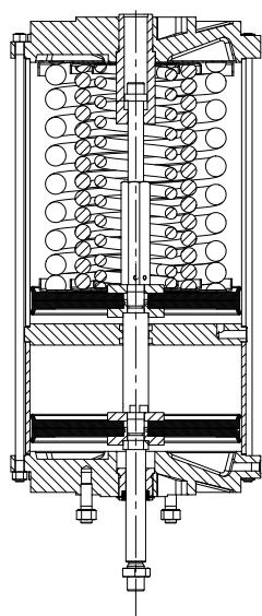
Type LAP-SF piston double
