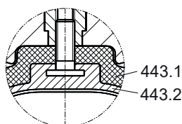
Variante membrane bipartie DN 250 - 300
