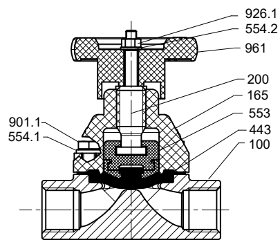
III. 1: Robinet à commande manuelle SISTO-16RGAMaXX
