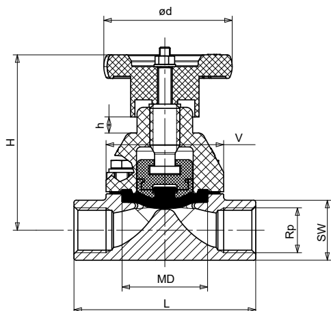
III. 2: Robinet à commande manuelle SISTO-16RGAMaXX
