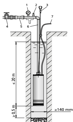
III. 3: Groupe motopompe suspendu à la tuyauterie de refoulement
