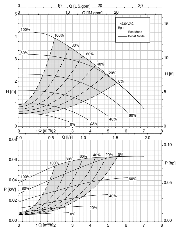
Calio 25-60 fonct. boucle ouverte, Eco-Mode
