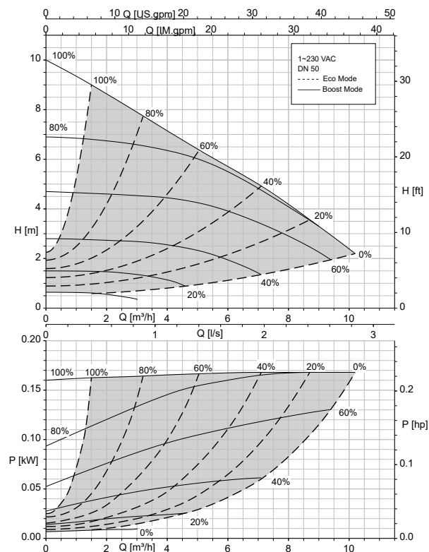
Calio 50-100 fonct. boucle ouverte, Eco-Mode
