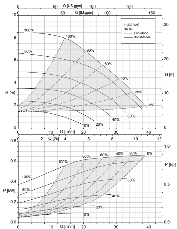
Calio 80-80 fonct. boucle ouverte, Eco-Mode
