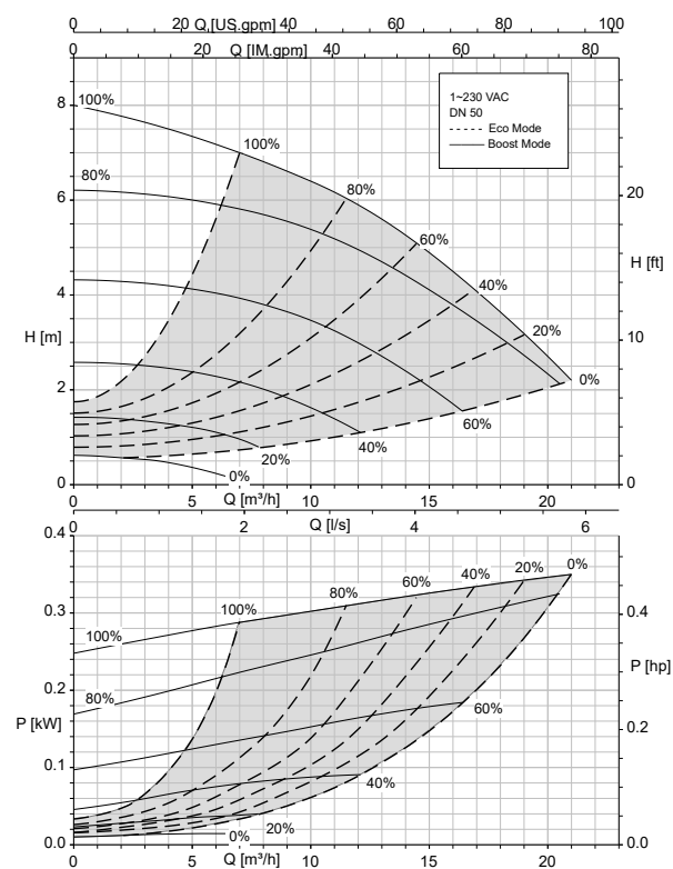
Calio 50-80 fonct. boucle ouverte, Eco-Mode
