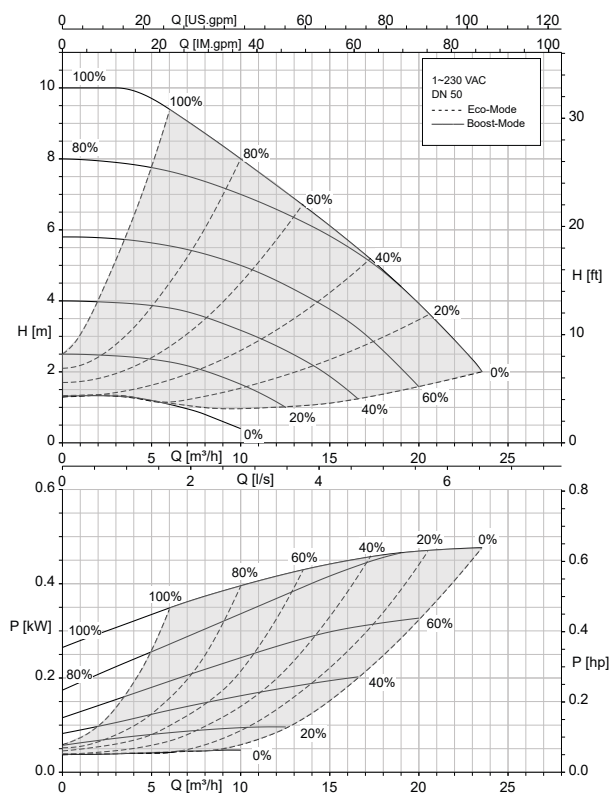
Calio 50-100 fonct. boucle ouverte, Eco-Mode
