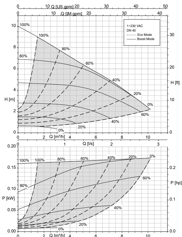
Calio 40-90 fonct. boucle ouverte, Eco-Mode
