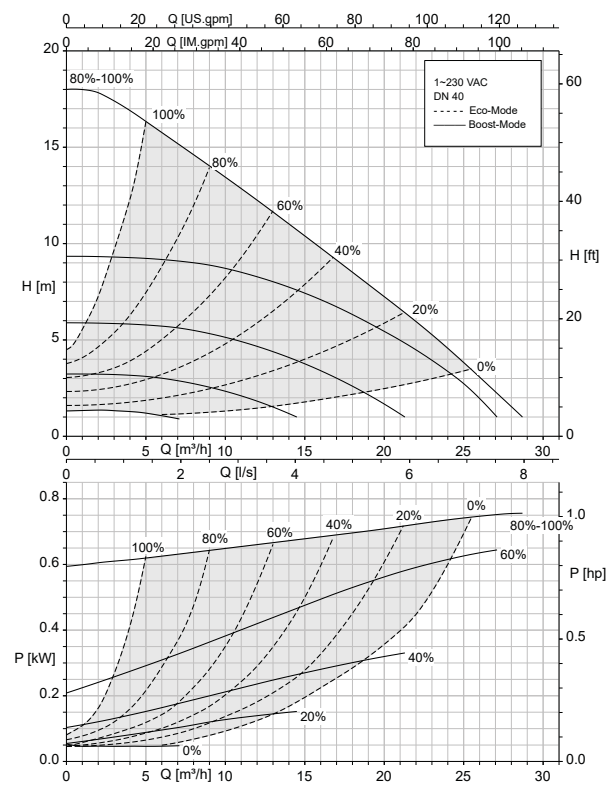
Calio 50-40 fonct. boucle ouverte, Eco-Mode
