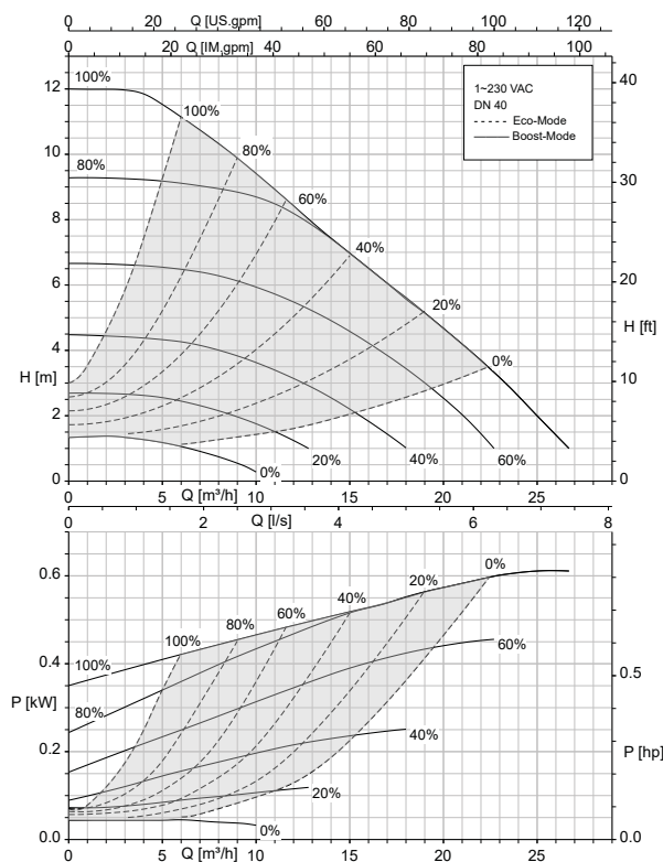
Calio 40-120 fonct. boucle ouverte, Eco-Mode
