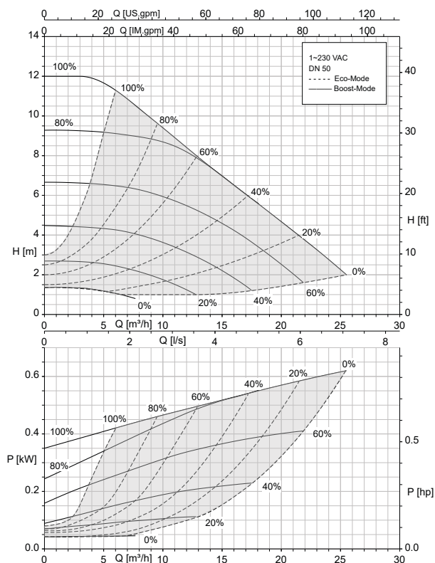
Calio 50-150 fonct. boucle ouverte, Eco-Mode
