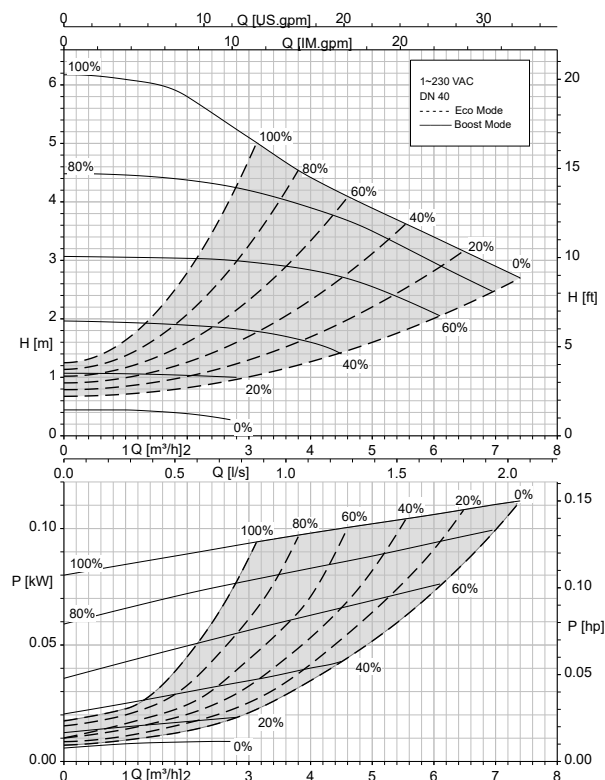
Calio 40-70 fonct. boucle ouverte, Eco-Mode
