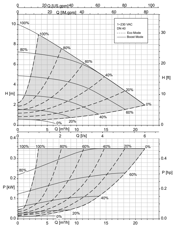
Calio 40-120 fonct. boucle ouverte, Eco-Mode
