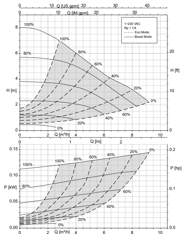
Calio 30-100 fonct. boucle ouverte, Eco-Mode
