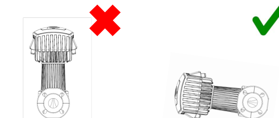
III. 3: Dépose sûre du groupe motopompe
