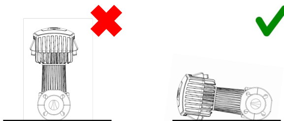
III. 6: Dépose sûre du groupe motopompe
