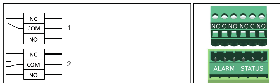
III. 10: Schéma de connexion report centralisé de défaut
