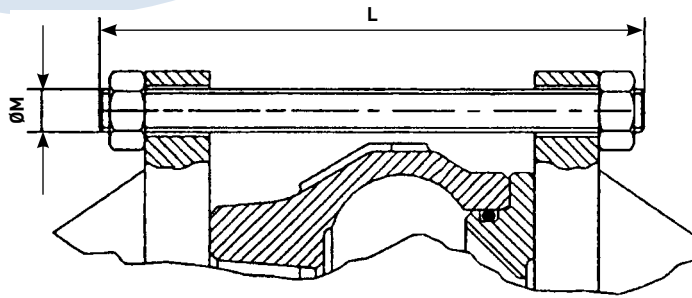
Montage entre brides DN 80 à DN 500
