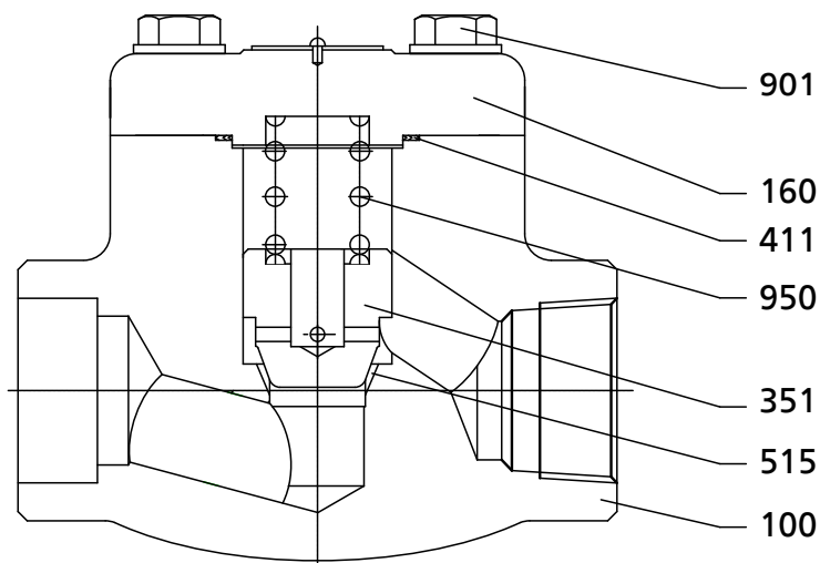
III. 1: Plan en coupe ECOLINE PTF 800
