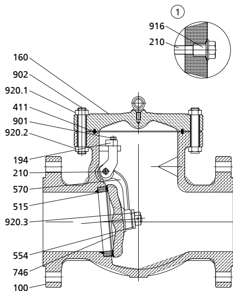
III. 1: Plan en coupe ECOLINE SCC 150-600
